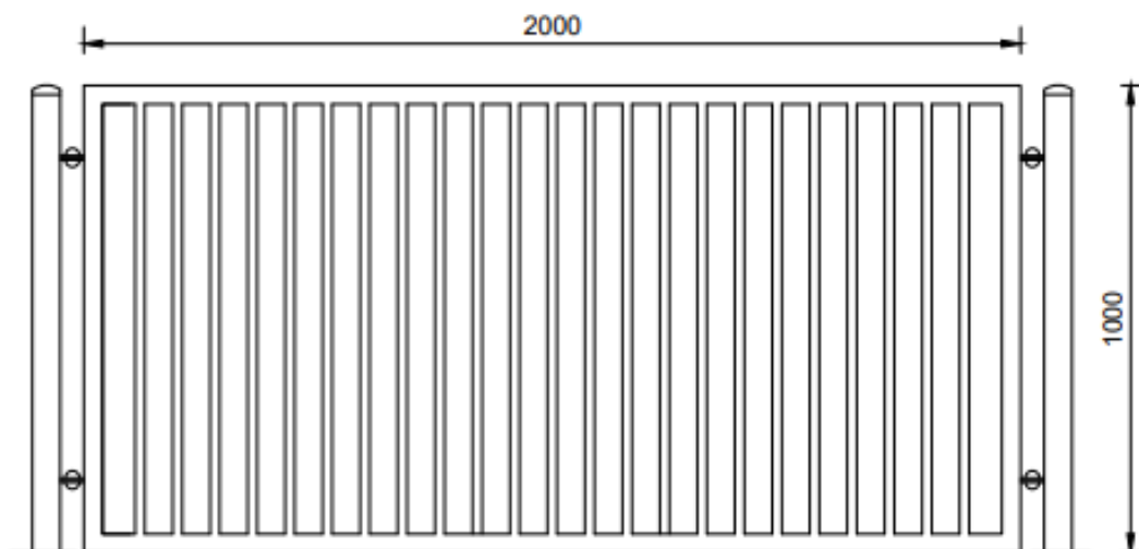
WIDOK Z FRONTU
